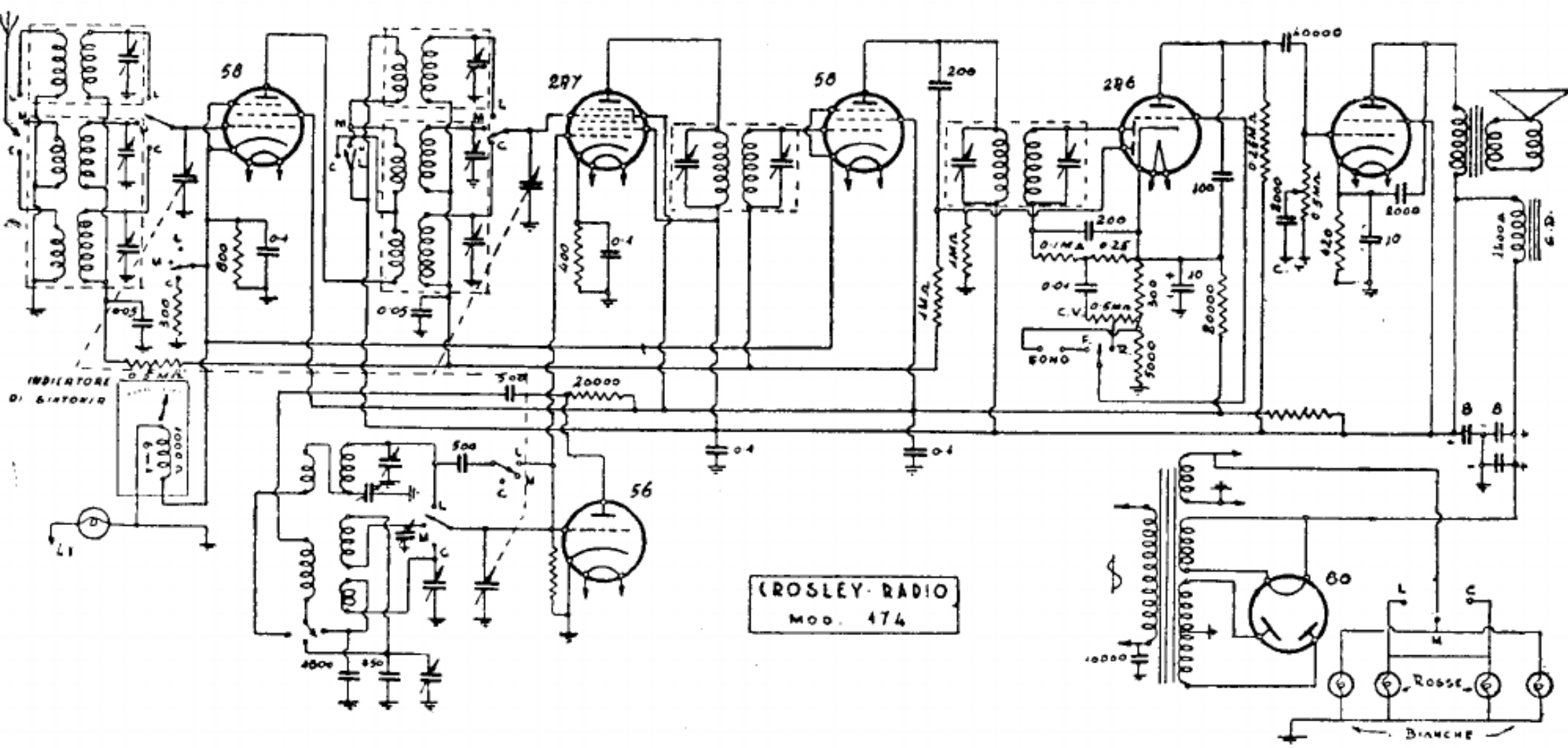
CROSLEY RADIO. — Modelli: « 174 A, 174 B e 174 C ». - Produzione 1934. - Media frequenza: 350 kc.
